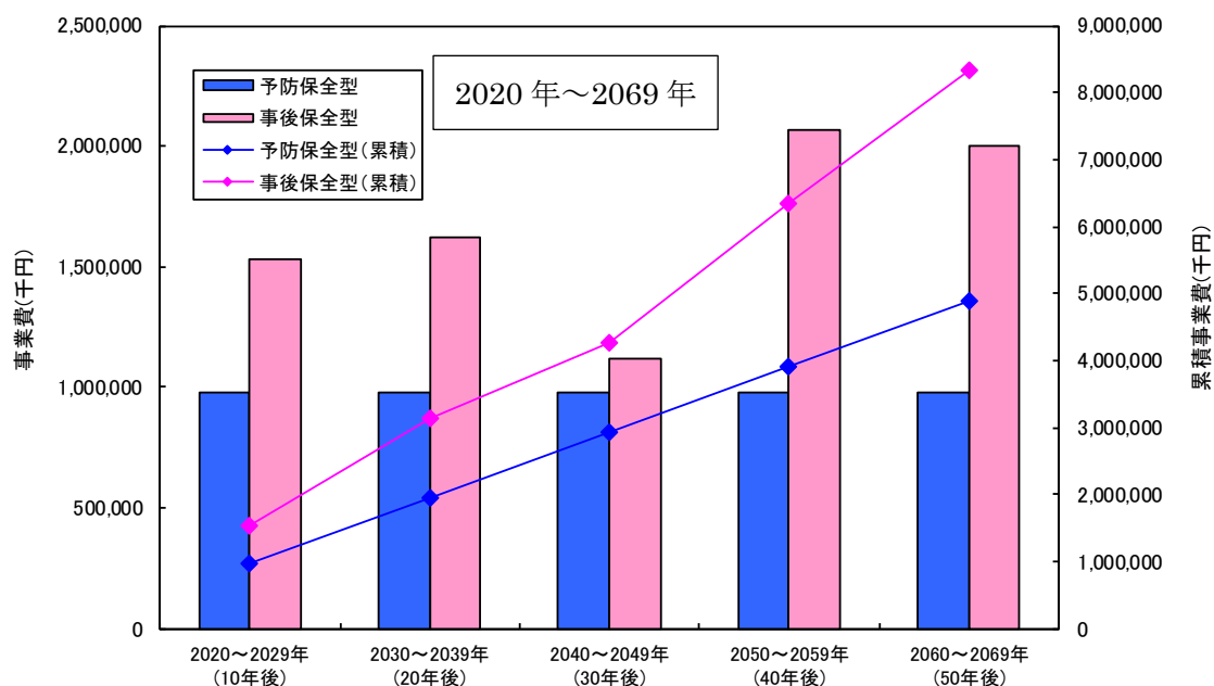
図－6.1 今後 50 年間ににおける予防保全型と事後保全型の累積予算比較
