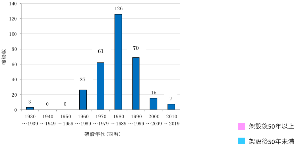
図－1.1 架設年別の内訳
