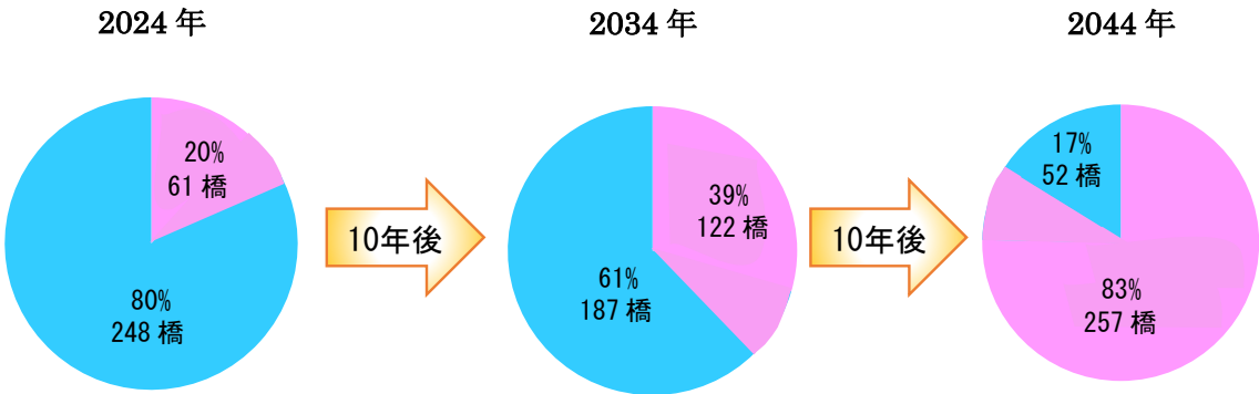
図－1.2 老朽化橋梁の推移
