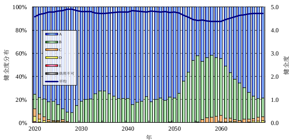
健全度分布の推移（部材別）
